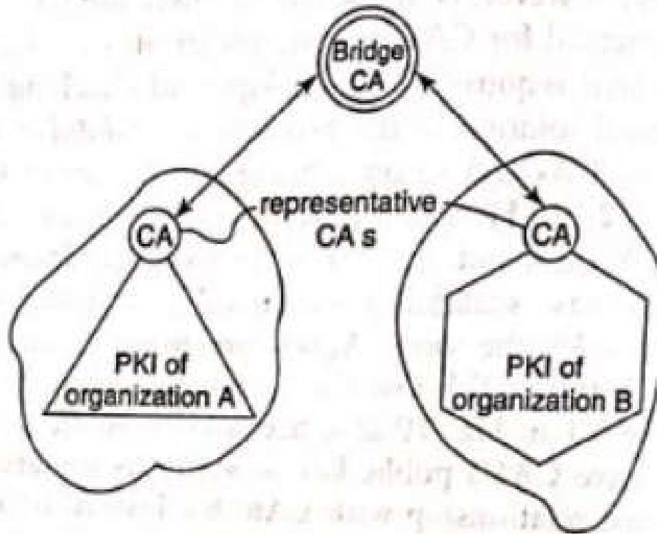
(d) Bridge-based PKI
